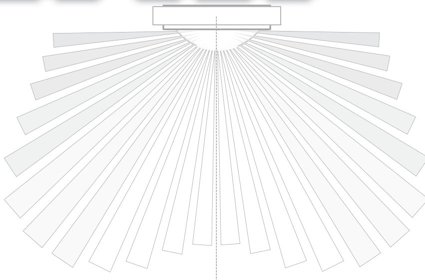
Variierbares Erfassungsfeld durch Abdeckfolie
